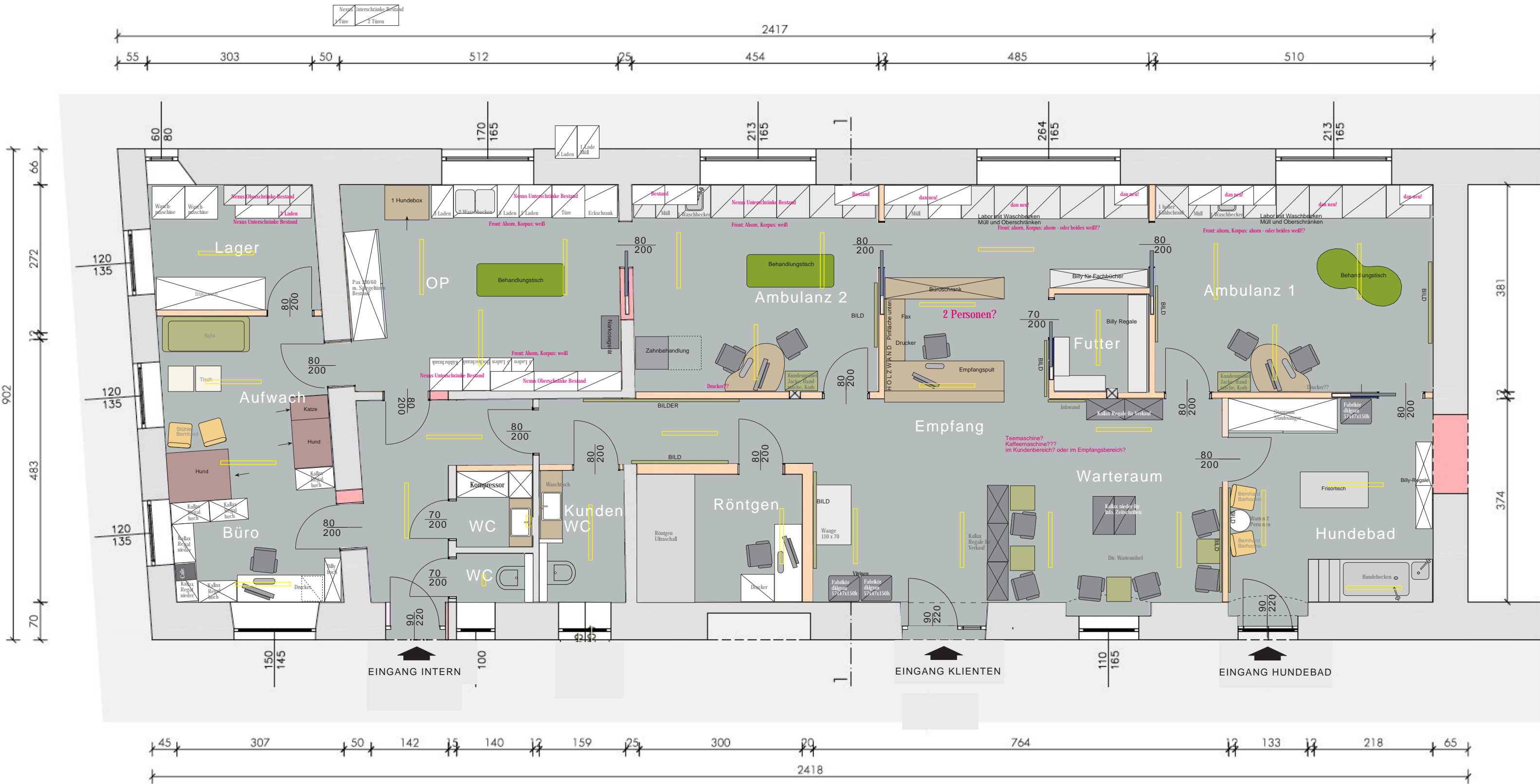
GRUNDRISS TIERARZTPRAXIS M 1:100 NTZFL 165,00 m 2
